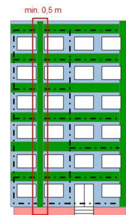
Obr. 7 – Svod
