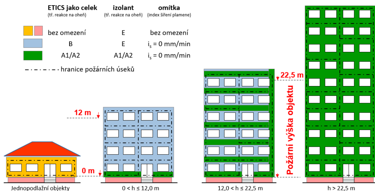
Obr. 1 – Schématické znázornění použití zateplovacích systémů
