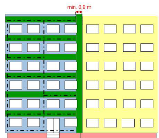
Obr. 3 – Sousední objekty
