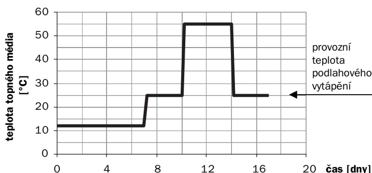
Náběhová křivka podlahového vytápění
