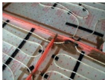
Prostup podlahového vytápění spárou
