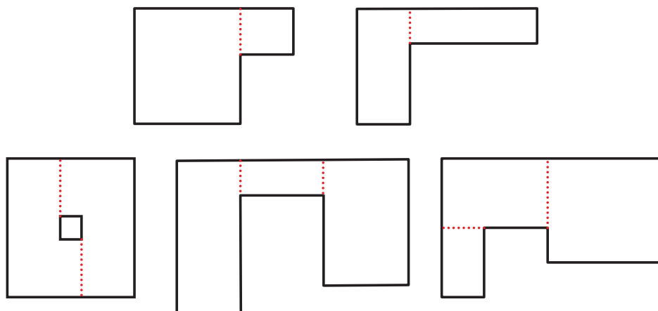
Možné rozdělení plochy mezilehlými spárami
