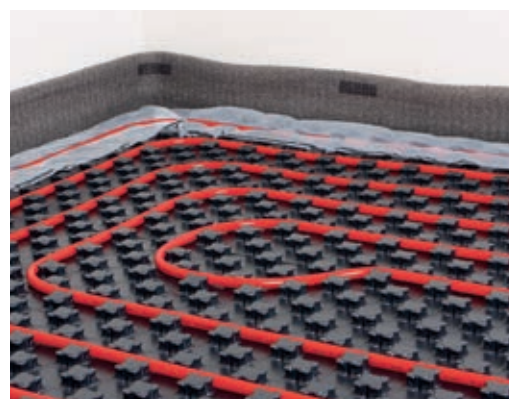
Systémová deska s podlahovým vytápěním
