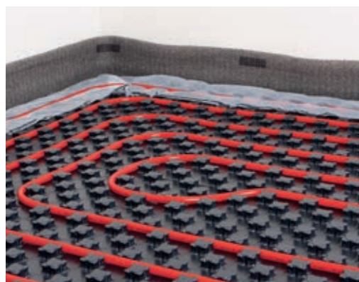
Montáž okrajové dilatační pásky, pokládka systému podlahového vytápění
