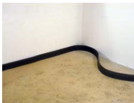
Osazení okrajové dilatační pásky
