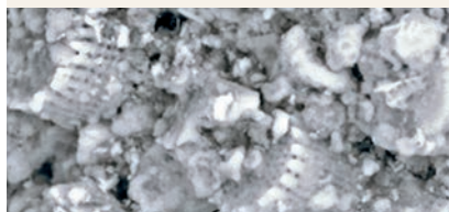
Mikroskopický snímek povrchu omítky Baumit StarTop s jeho korálovým tvarem mikroplyniva
