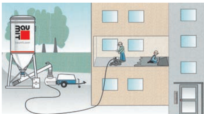
Obrázek 17: Cementové potěry
