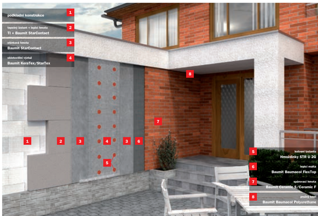
Obrázek 7: Zateplovací systém Baumit Kera
