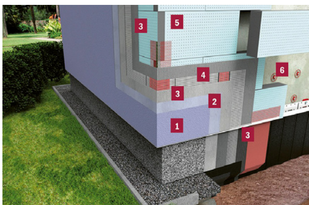
Baumit open – řez systémem zateplení
