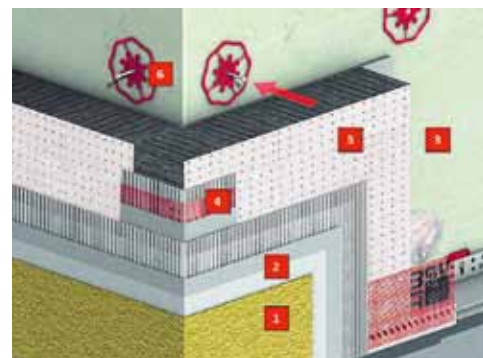
Baumit open – řez systémem zateplení
