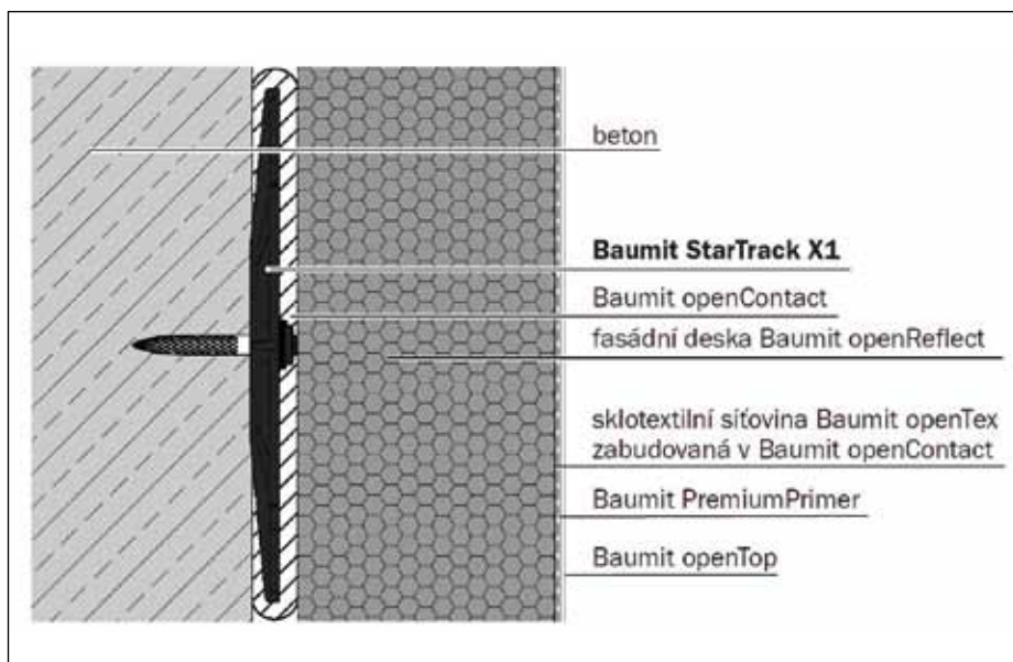
Řez konstrukcí – vrstvy
