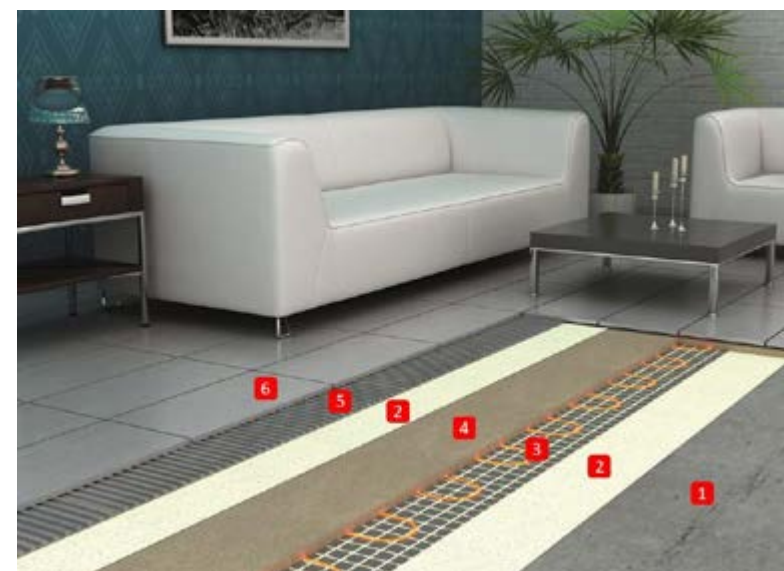
Příklad skladby konstrukce při použití podlahového vytápění s elektrickým odporovým drátem: 1. Podkladní beton, 2. Baunit SuperPrimer – základní nátěr, 3. Elektrický odporový drát – podlahové vytápění, 4. Baunit Nivello Quattro – samonivelační sádrová stěrka, 5. Baunit Baumacol FlexTop / FlexUni – lepicí malta, 6. Baunit Baumacol PremiumFuge – spárovací hmota
