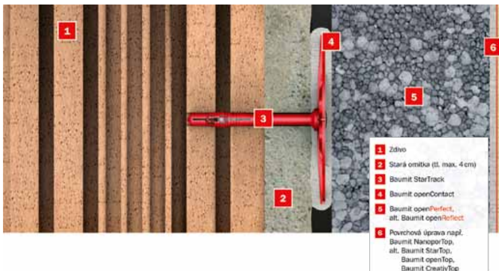
Skladba zateplovacího systému ETICS Baumit open
