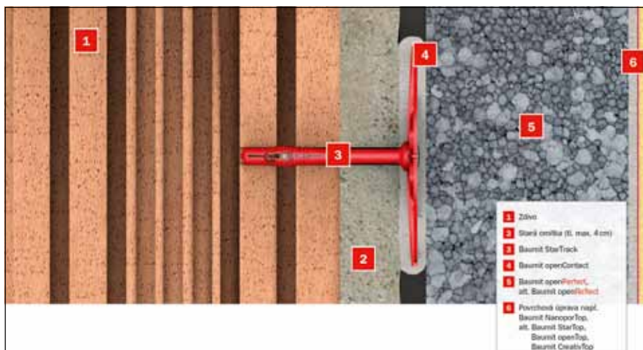
Skladba zatepovacího systému ETICS Baumit open
