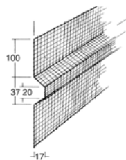
Profil typ II
